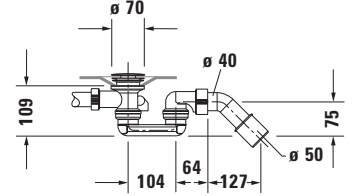
Küvet için sifon # 700476
