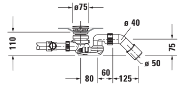
Masajlı küvet için sifon # 760476
