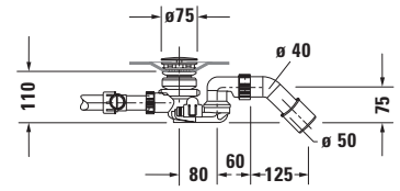
Masajlı küvet için sifon # 760478
