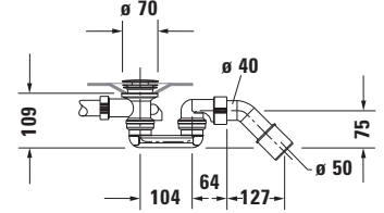
Küvet için sifon # 700478
