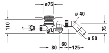
Masajlı küvet için sifon # 760475
