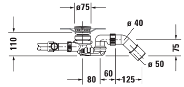
Masajlı küvet için sifon # 760472
