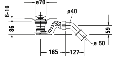
Küvet için sifon # 700486
