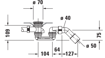
Küvet için sifon # 700475
