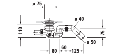
Masajlı küvet için tabandan su girişli sifon # 760426
