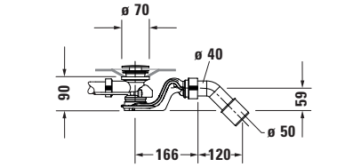
Masajlı küvet için sifon # 760426
