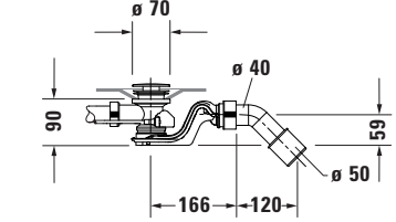
Düz Küvet için sifon # 700429
