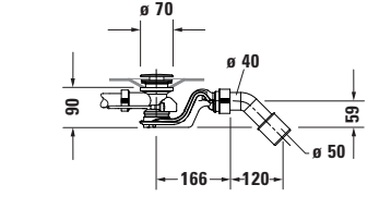
Masajlı küvet için sifon # 760429
