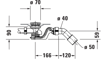
Düz Küvet için sifon # 700427
