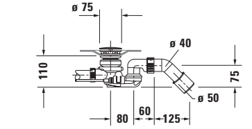
Küvet için tabandan su girişli sifon # 700428
