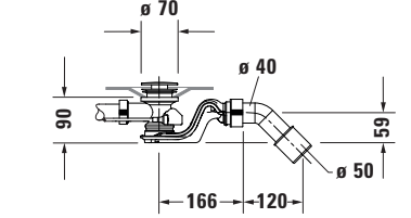
Düz Küvet için sifon # 700426
