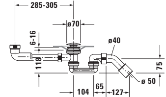
Düz Küvet için sifon # 700460
