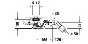
Masajlı küvet için sifon # 760428
