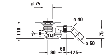
Masajlı küvet için tabandan su girişli sifon # 760428
