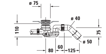
Masajlı küvet için tabandan su girişli sifon # 760429
