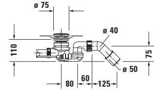
Küvet için tabandan su girişli sifon # 700427
