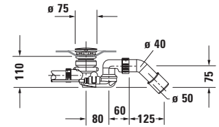
Masajlı küvet için tabandan su girişli sifon # 760427
