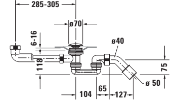
Düz Küvet için sifon # 700430
