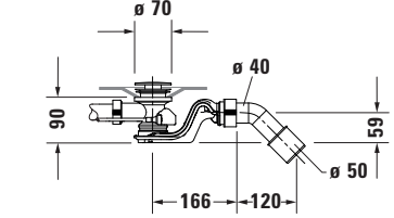
Düz Küvet için sifon # 700428
