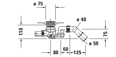
Küvet için tabandan su girişli sifon # 700426
