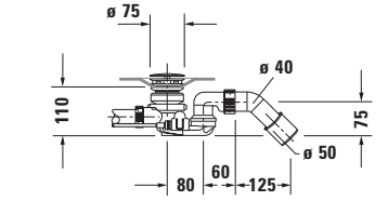
Küvet için tabandan su girişli sifon # 700429
