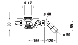
Masajlı küvet için sifon # 760427
